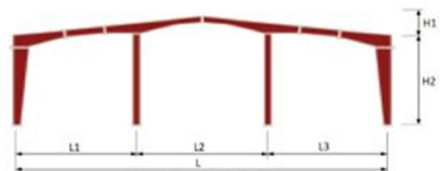
Khung thép điển hình 3 nhíp
