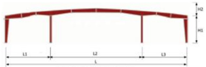
Khung thép định hình 3 nhíp
